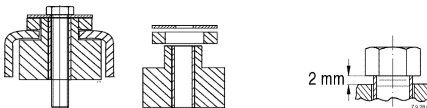
Виброопоры одиночного компрессора
