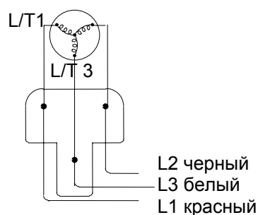
рис. 7 Контакты компрессора
