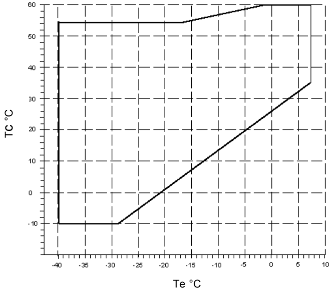
ZF24 до ZF48K4E
