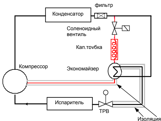
Рис.3 Впрыск пара
