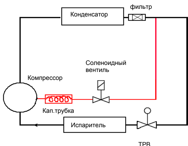
Рис.2 Впрыск жидкости
