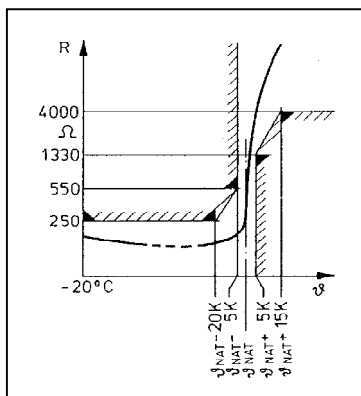
рис 8: Сопротивление термистора
