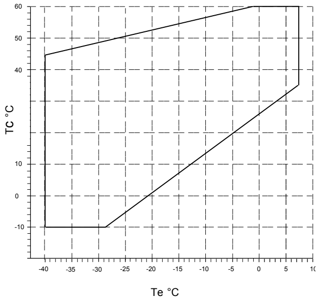
ZF24K4E до ZF48K4E С экономайзером
