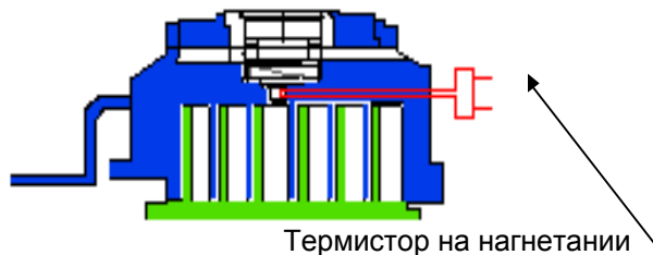
рис. 5 расположение термистора на нагнетании
