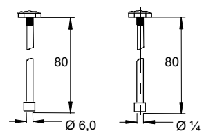
U/X 6 мм / 1/4" ODF пайка трубка длиной 80 мм
